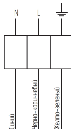
Рис. 11. Схема подключения изделия к сети 220В
